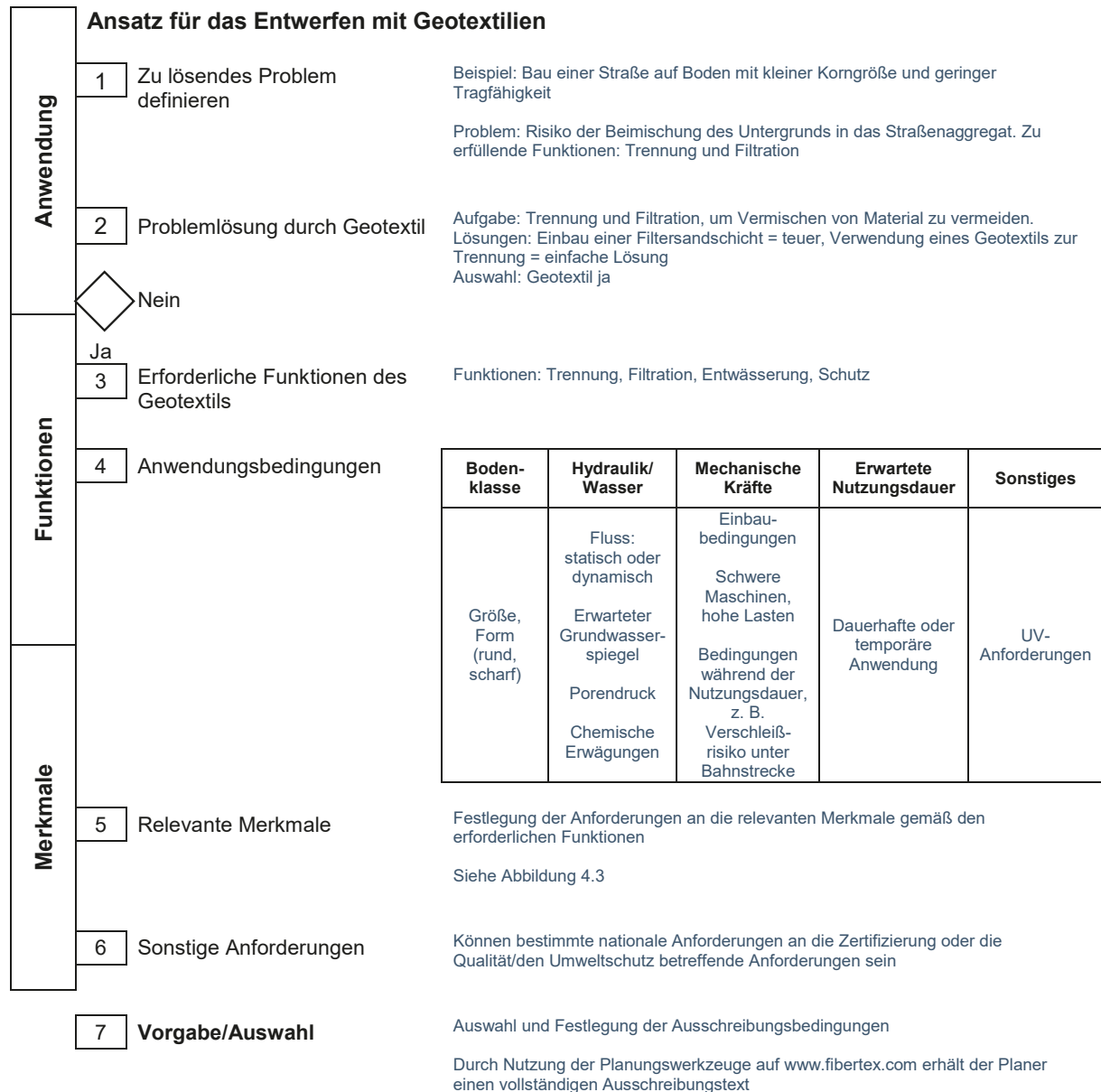
Abbildung 4.4 Ansatz für das Entwerfen mit Geotextilien
