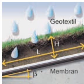
Abbildung 5.17 Entwässerung auf einem geneigten Dachgarten
