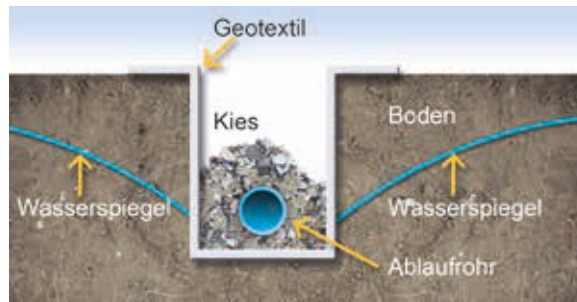
Abbildung 5.10: Verlegung in Entwässerungsgräben
