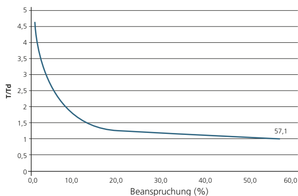
Abbildung 6.6: Erwartetes erforderliches Belastungsniveau in praktischen Anwendungen
