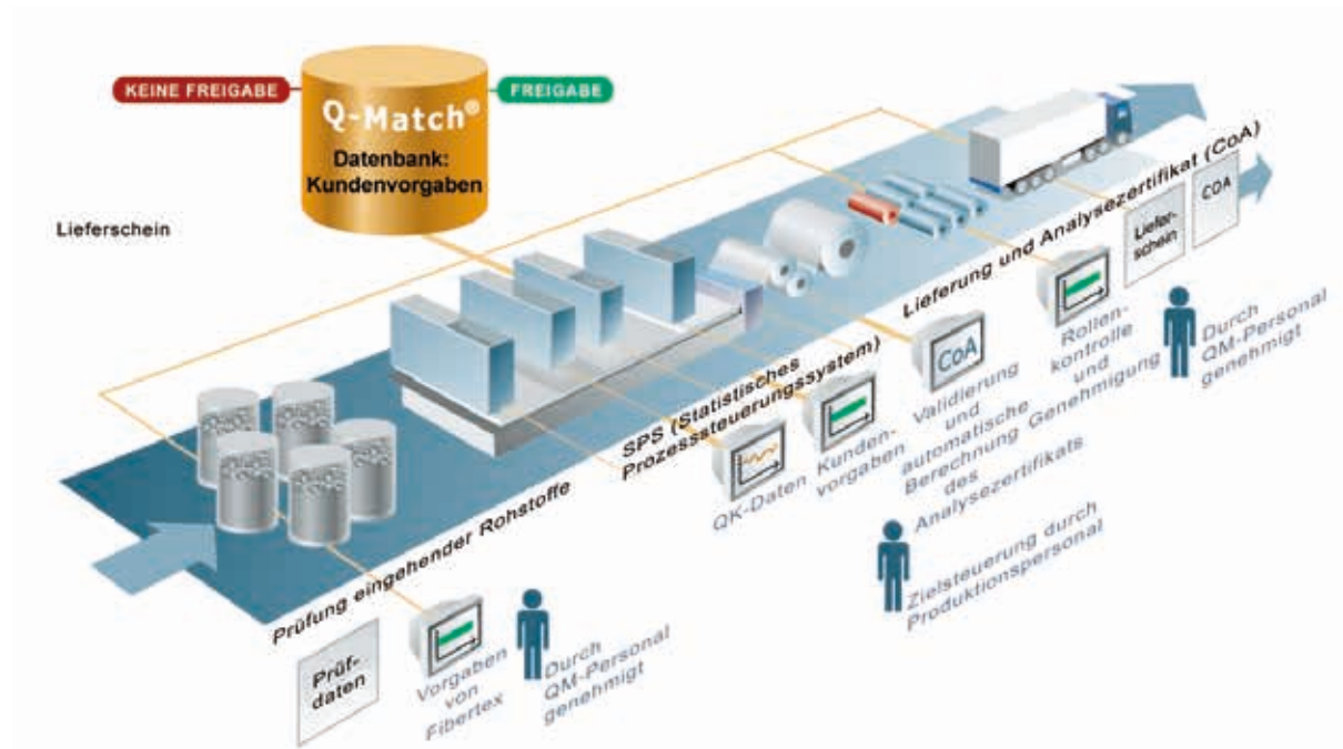
Abbildung 3.4 Q-Match – das vollständig digital integrierte Qualitätsmanagementsystem von Fibertex
