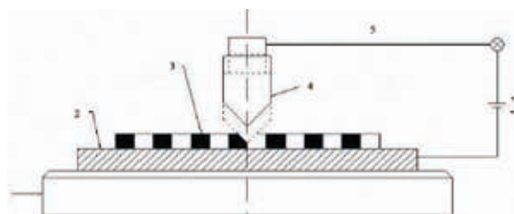
Abbildung 5.20 Prinzipieller Aufbau der Schutzwirksamkeitsprüfung nach EN 13719. /EN 13719/
