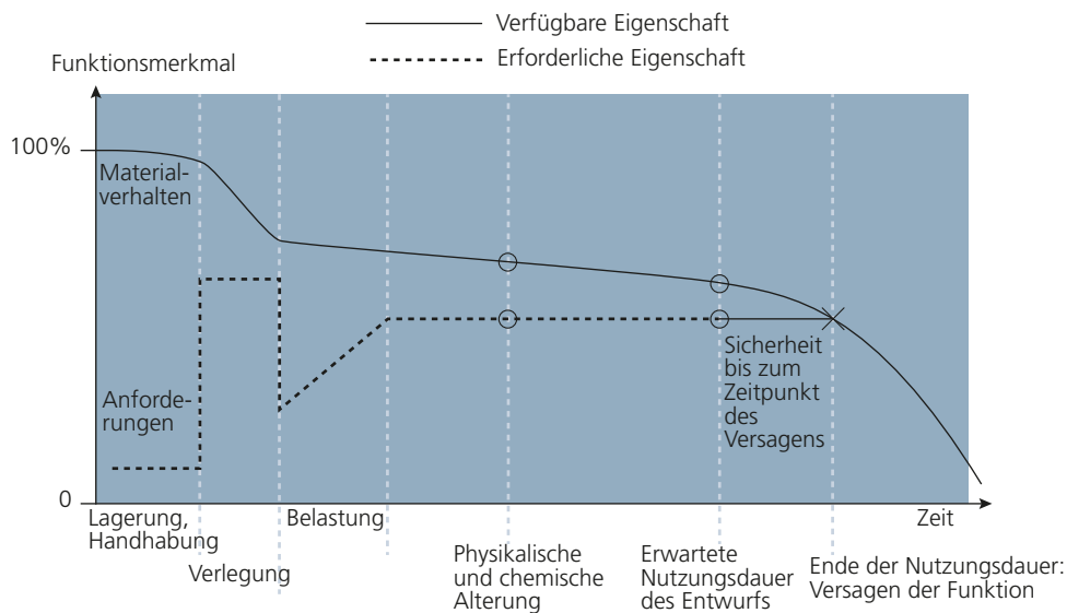
Abbildung 6.1 Typische verfügbare und erforderliche Werte einer Funktionseigenschaft im zeitlichen Verlauf /EN 13434/
