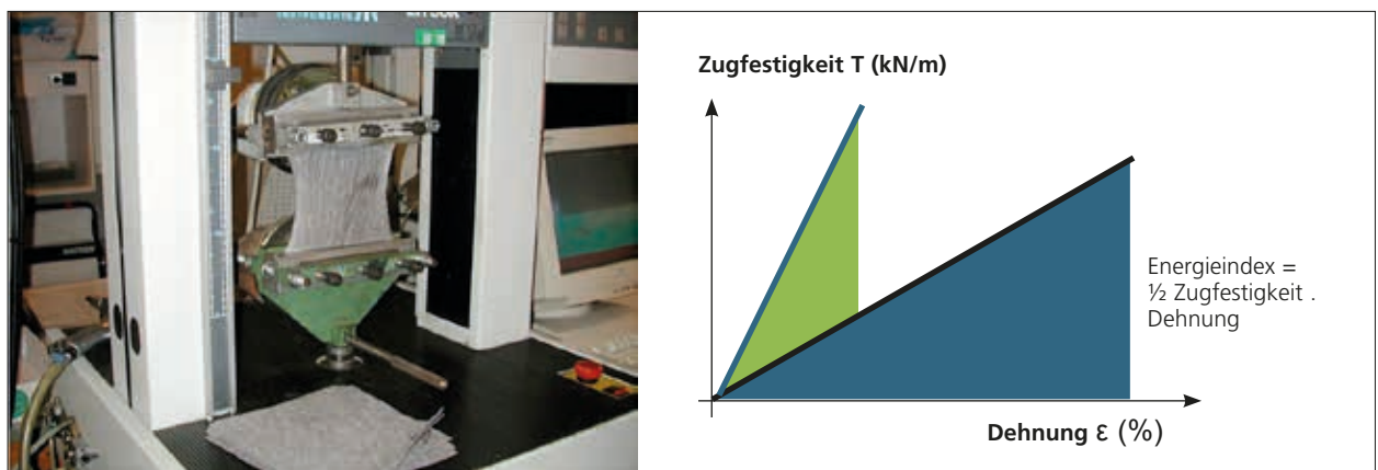
Abbildung 6.3 Ein steifes Geotextil benötigt eine höhere Zugfestigkeit als ein Geotextil mit stärkerer Dehnung, um den gleichen Energieindex zu erreichen
