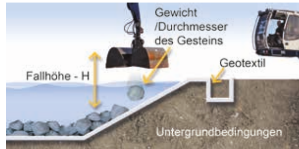
Abbildung 6.10 Beispiel eines Wasserbauwerks – Verlegung und Entwurf
