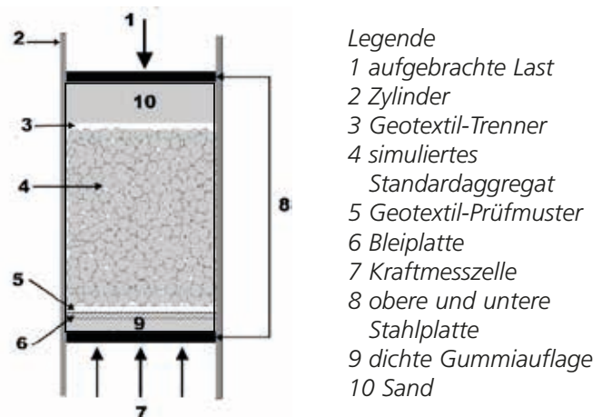
Abbildung 5.20 Prinzipieller Aufbau der Schutzwirksamkeitsprüfung nach EN 13719. /EN 13719/
