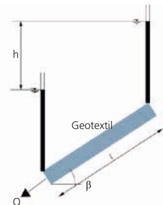
Abbildung 5.16 Berechnung des hydraulischen Gefälles für geneigte Abläufe
