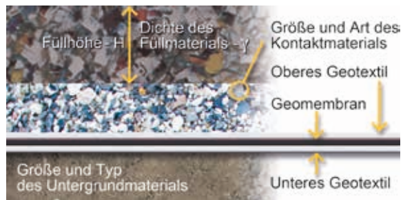
Abbildung 5.23 Geotextil zum Schutz in einer Abfallbeseitigungsanlage
