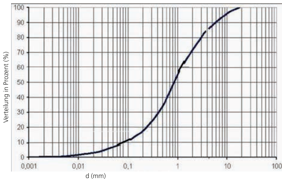
Abbildung 5.11 Korngrößenkurve für zu filternden Boden
