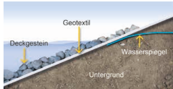
Abbildung 5.12 Küstenschutzbauwerk mit Deckgestein und Geotextil
