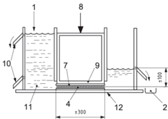
Abbildung 5.14 Prinzipieller Aufbau zur Prüfung des Wasserableitvermögens in der Ebene nach EN ISO 12958./EN ISO 12958/
