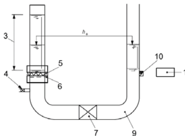
Abbildung 5.7 Prinzipieller Aufbau zur Geschwindigkeitsindexprüfung nach EN ISO 11058 unter Anwendung der Methode der fallenden Druckhöhe. IEN ISO 11058/
