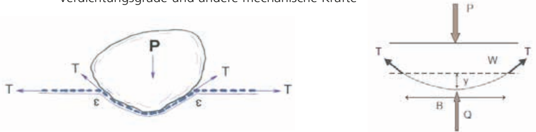
Abbildung 6.5 Realistische Standortbedingungen und vereinfachtes Modell zur Spannungs-/Dehnungsbewertung
