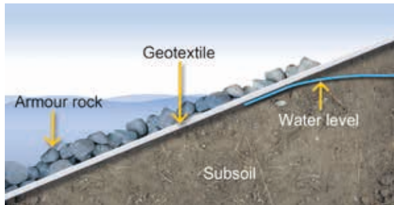
Schéma 5.12: Protection côtière utilisant des enrochements et du géotextile
