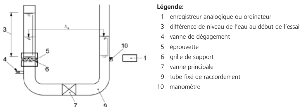
Figure 5.5: Principe de l'essai de l'indice de vitesse (NF EN ISO 11058) selon la méthode de la chute d'eau
