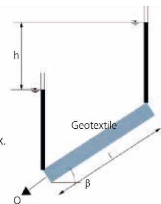
Figure 5.16: Calcul du gradient hydraulique pour les drains inclinés
