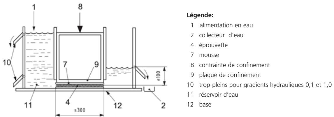
Figure 5.14: Fonctionnement principal de l'essai de capacité de débit dans le plan suivant la norme NF EN ISO 12958.
