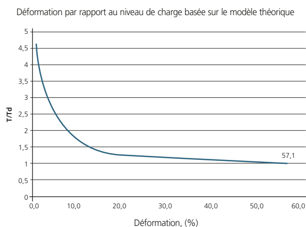
Figure 6.6: Niveau attendu de la déformation requise dans les ouvrages courants
