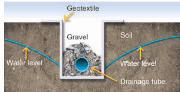
Schéma 5.10: Mise en œuvre d'une tranchée drainante
