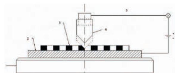
Figure 5.21: Fonctionnement principal de l'essai de résistance au poinçonnement pyramidal suivant la norme NF EN 14574
