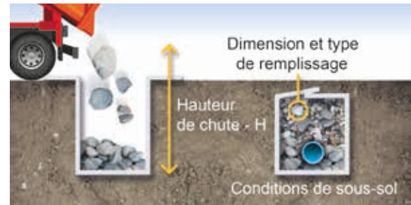
Figure 6.7: Exemple de mise en œuvre d'une tranchée drainante
