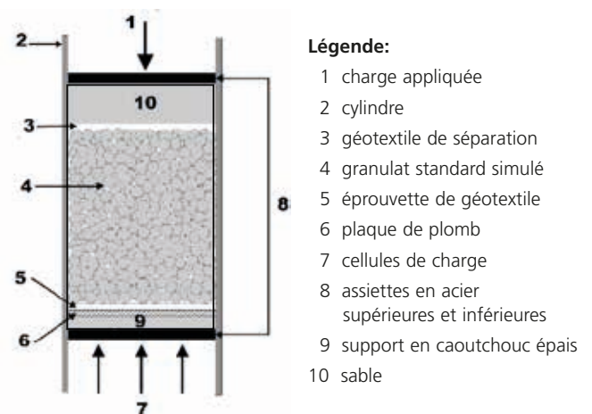
Figure : 5.20: Fonctionnement principal de l'essai d'efficacité de protection suivant la norme NF EN13719.
