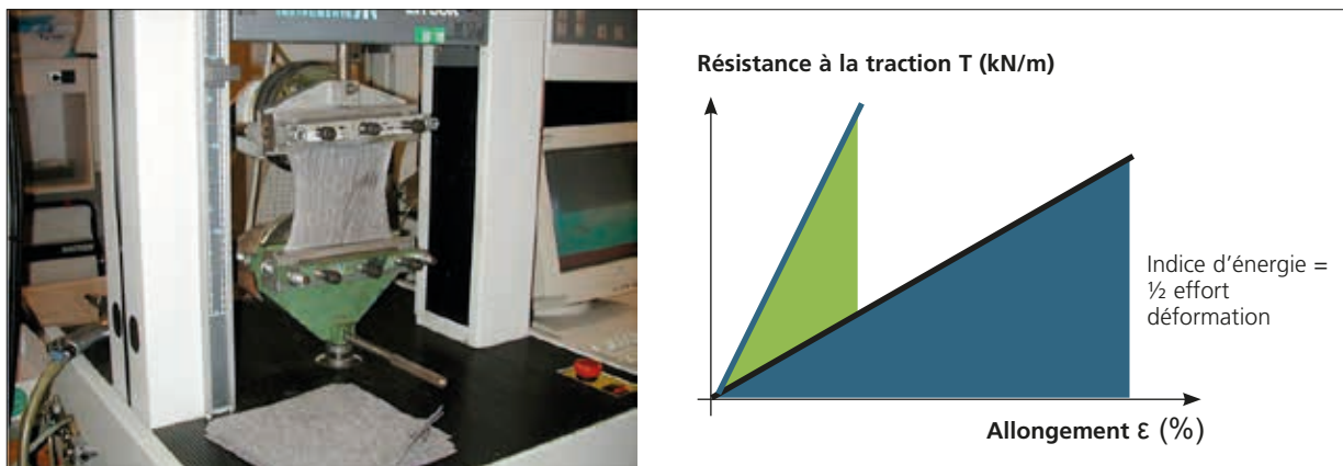
Figure 6.3: Un géotextile peu déformable nécessite davantage de résistance à la traction qu'un géotextile avec un allongement plus élevé pour atteindre la même absorption d'énergie.
