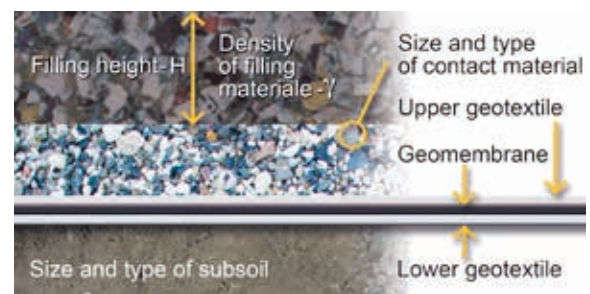
Schéma 5.23: Géotextile utilisé en protection dans une installation de stockage de déchets
