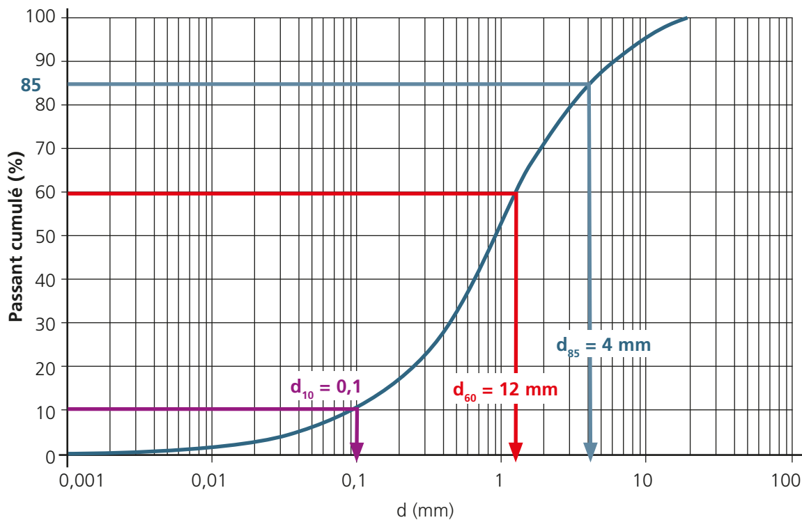
Figure 5.8: Exemple de sol continu et étalé ( C_u=12 )
