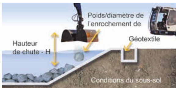
Figure 6.11: Exemple d'une structure hydraulique – conception et mise en œuvre
