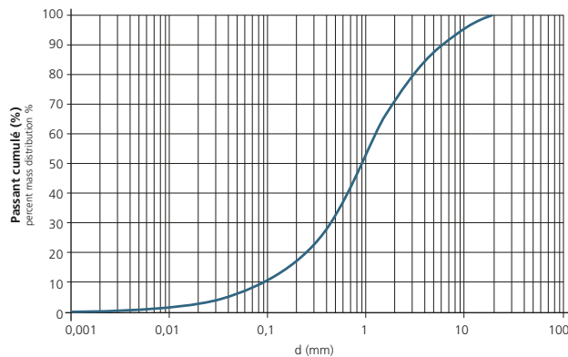
Figure 5.11: Courbe granulométrique du sol à filtrer
