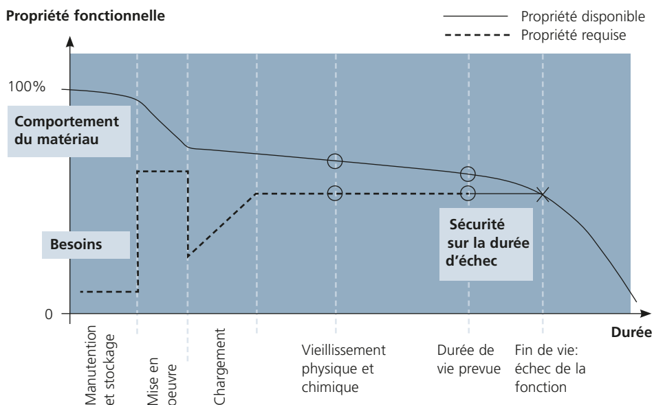
Figure 6.1: Valeurs types disponibles et requises d'une propriété fonctionnelle en fonction de la durée (EN 13434)
